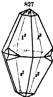
Calcite.
